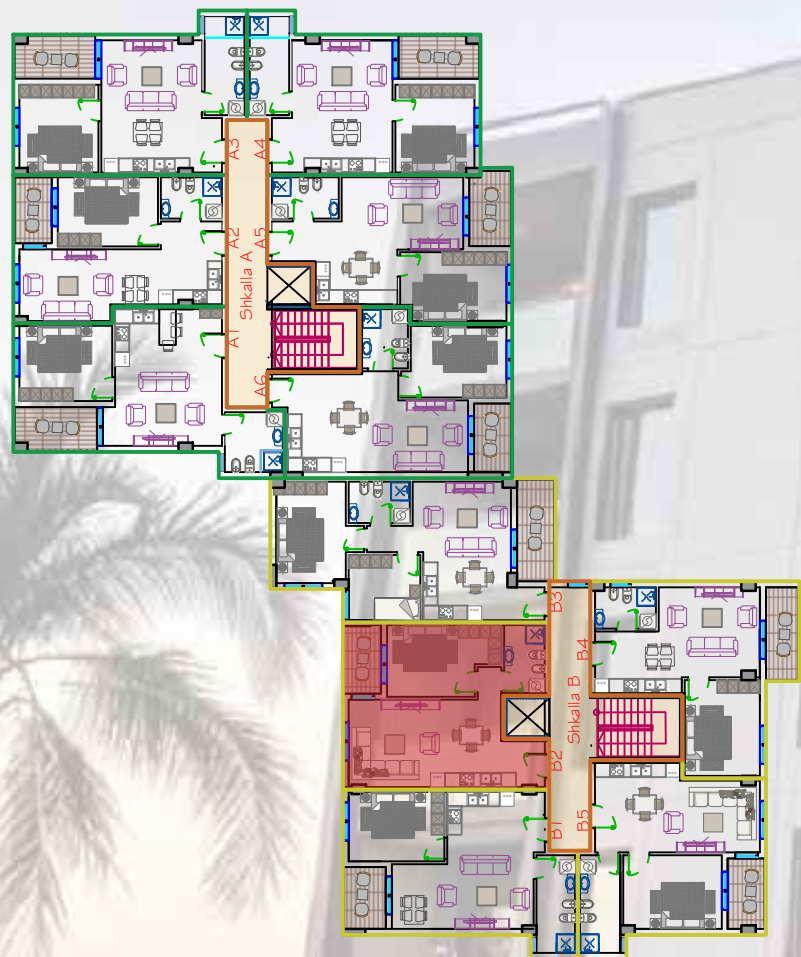
PLANIMETRIA E OBJEKTIT
